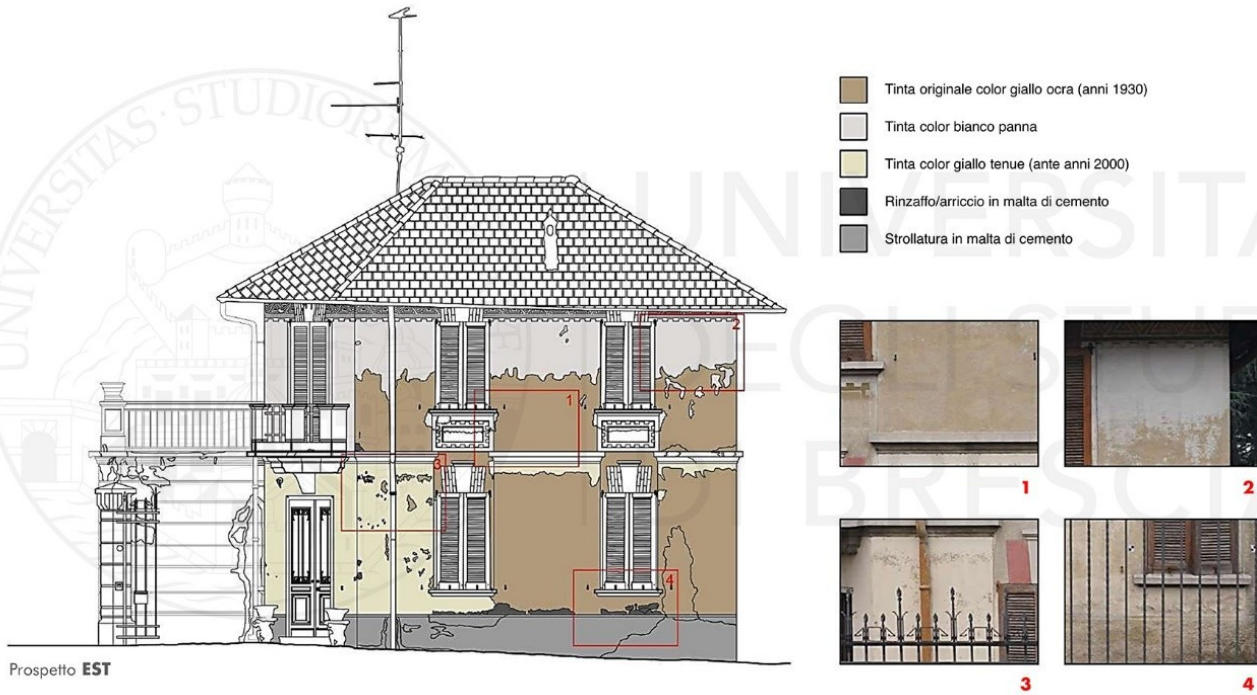
tavola del rilievo materico che evidenzia la stratificazione di intonaci e tinte - prospetto est
